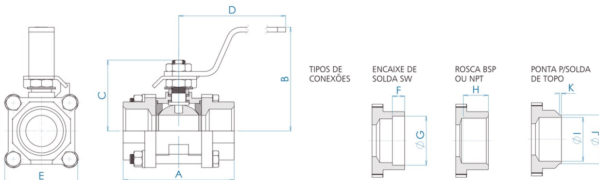
Desenho dimensional e tipos de conexão (cotas conforme tabela de especificações)
